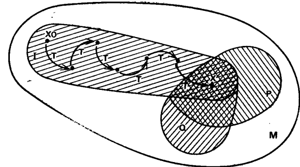
Рис. 4.3. Схема проектирования цикла с помощью инварианта
