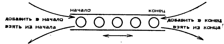
Рис. 7.3. Дек
