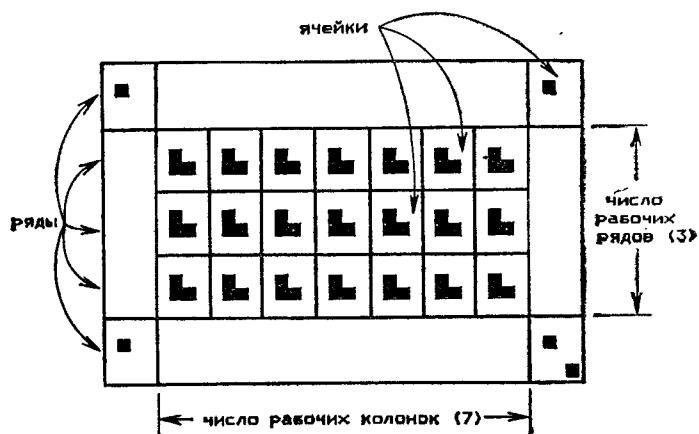
Рис. 8.2. Сито
