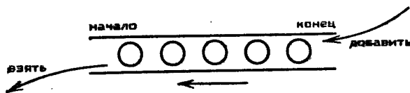
Рис. 7.2. Очередь
