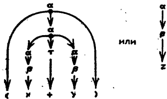
Рис. 10.1. Деревья вывода для формул (x + y) и z
