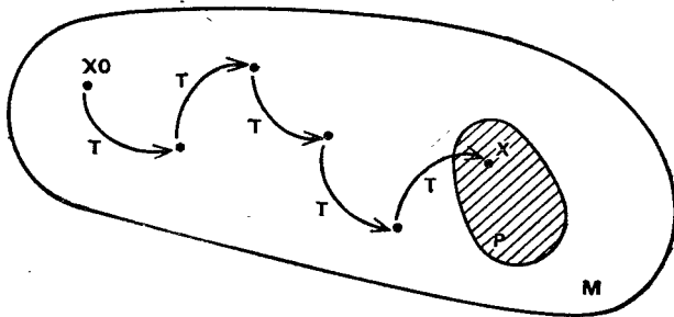
Рис. 4.2. Метод итераций
