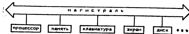
Рис. 19.1. Общая схема ЭВМ архитектуры PDP-11
