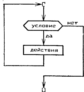
Рис. 2.4. Конструкция цикл — пока — выполнять — конец цикла
